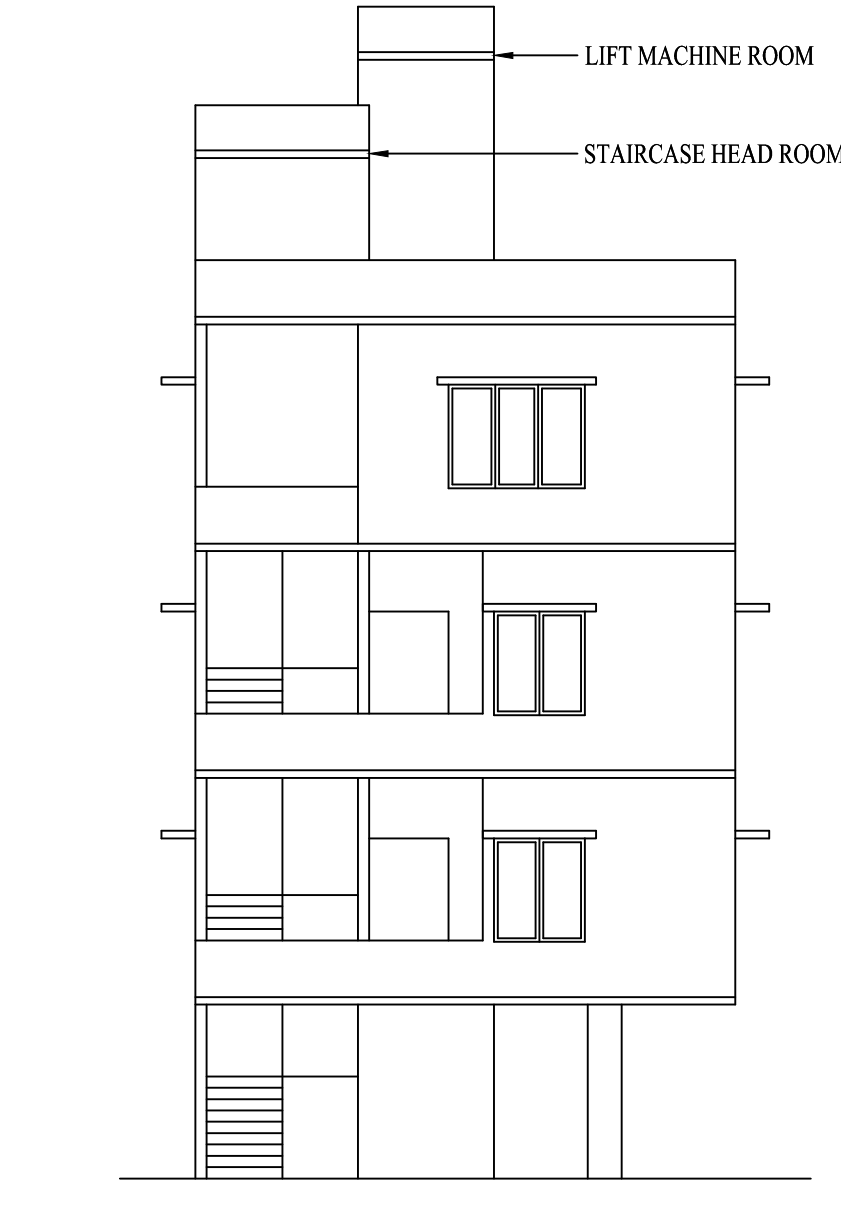
ELEVATION
